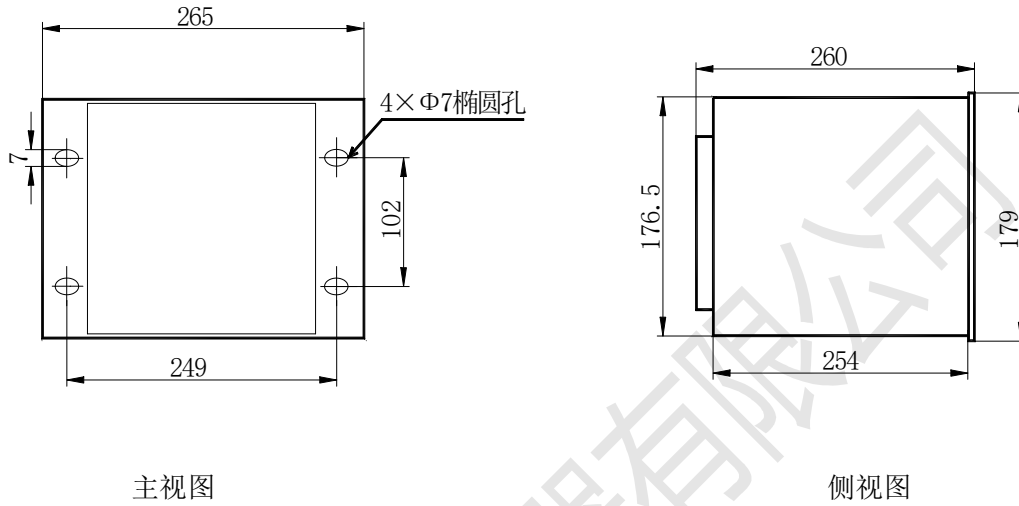
机箱外形尺寸图
