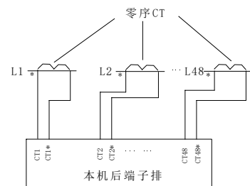
零序电流互感器接入方法
